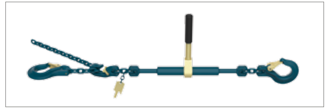
Bild 2: MAXNORM 12 Zurrkette einseitig mit Gabelkopfhaken und andererseits Verkürzungshaken und Hakenkette
