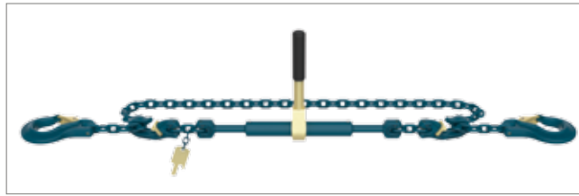
Bild 1: MAXNORM 12 Zurrkette beidseitig mit Verkürzungshaken und Hakenkette
