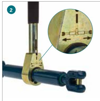
Bild 1: Spannen
